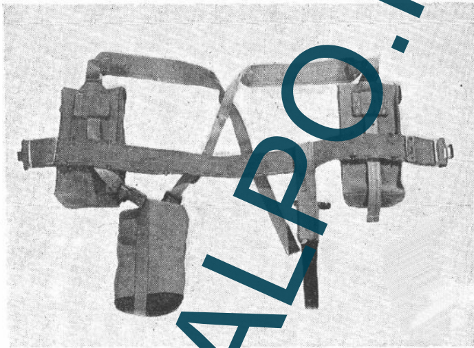
2 a serie di equipaggiamento.
